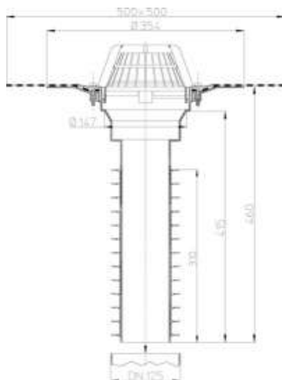
Рис. 3. Кровельная воронка HL69H/2.
