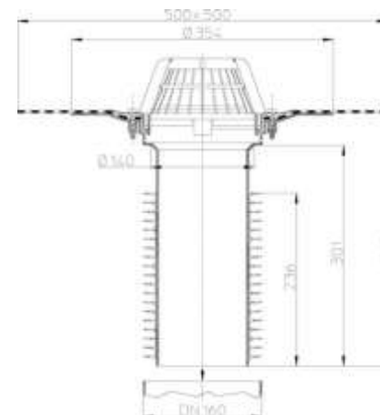
Рис. 4. Кровельная воронка HL69H/5.
